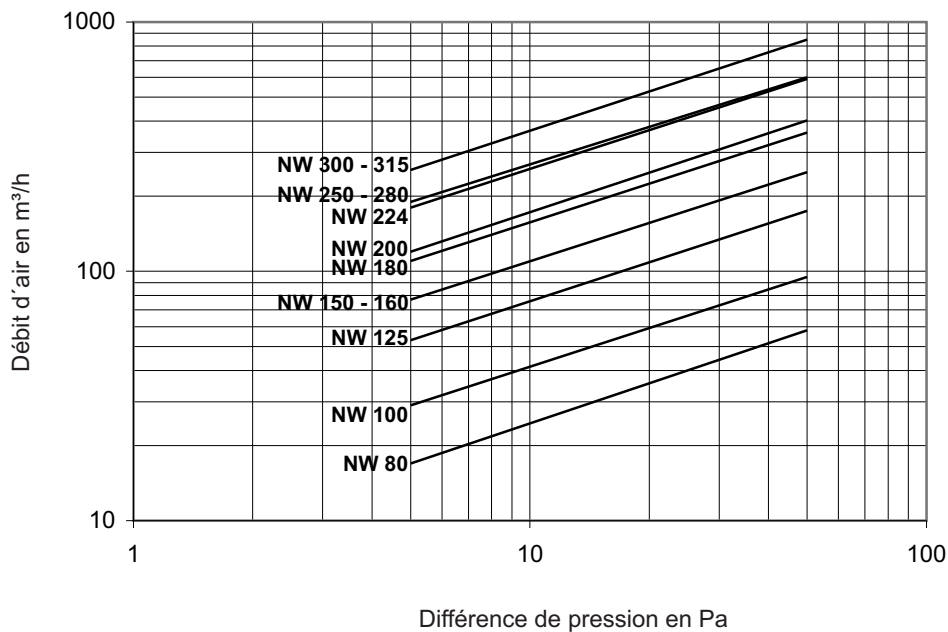
Diagramm1: perte de charge de la grille pare pluie en air aspiré
