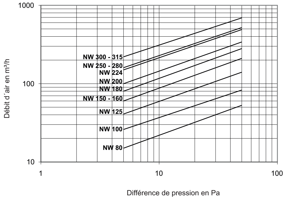
Diagramm1: perte de charge de la grille pare pluie en air extrait
