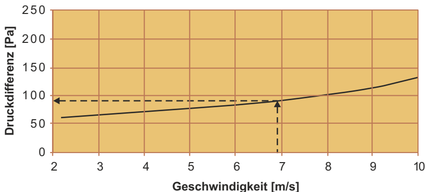
Diagramm 2: Statische Mindestansprechdruckdifferenz am Volumenstromregler
