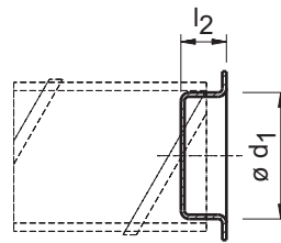
Anwendung 2 Rohrverbindung
